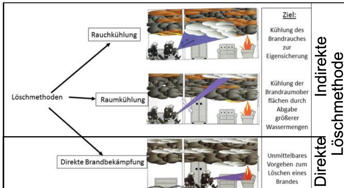
Abbildung 6 - Übersicht der Löschmethoden nach DIN 14011. (Grafik: Fuchs/ Südmersen, ecomed-Storck GmbH)
