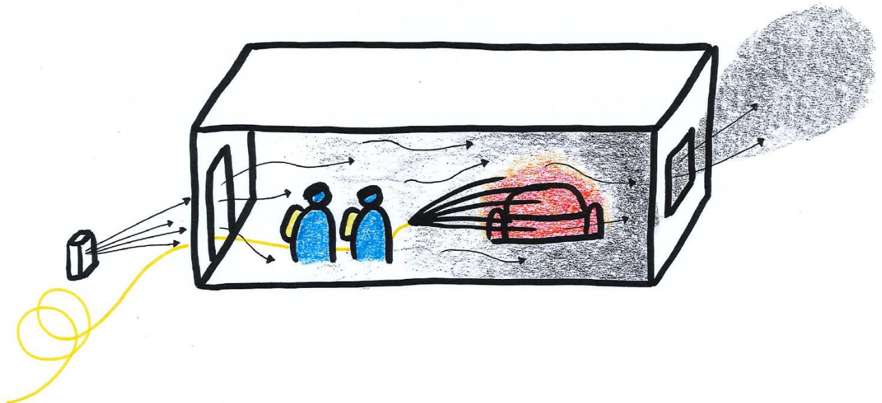
Abbildung 31 - optimaler Fall einer taktischen Ventilation als Erstmaßnahme, die gesamte Rauchschicht schiebt sich vor dem Angriffstrupp zur Abluftöffnung, verringert hierbei Wärme, Atemgifte und Sichtbehinderung, so dass der Trupp effektiver vorgehen kann; Quelle: Stephanie Vöge IdF NRW
