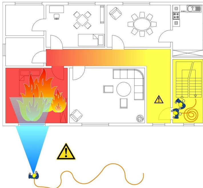
Abbildung 18 - Negative Verschiebung der Gefahrenbereiche bei offener Brandraumtür und offenem Fenster als Ventilationsöffnung durch Fensterimpuls mit Sprühstrahl von außen (Abdeckung der Ventilationsöffnung!), Jürgen Buil
